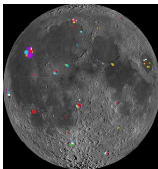
Рис. 3. Распределение КЛЯ на диске Луны по цветам
