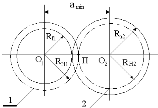
Рис. 1. Центроиды винтовых поверхностей резьбы (1) и червячной фрезы 2:
