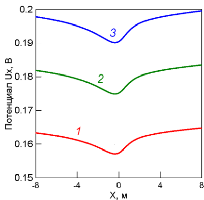
Рис. 4. Потенциал в верхнем слое грунта в нормальном сечении к оси трубы
