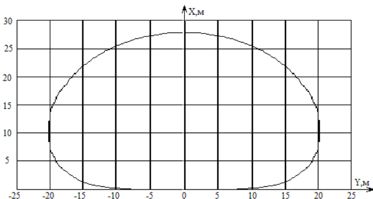
Рис. 3. Линия возможного положения рамки в системе координат ОХУ при наличии аддитивной погрешности, равной 1 % от значения напряженности при y = 10 м, и базе измерения 2a = 2 м
